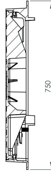
A-A (1 : 10)
