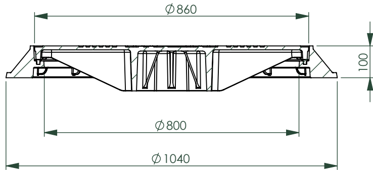
B-B (1 : 12)
