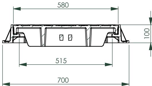
B-B (1 : 12)
