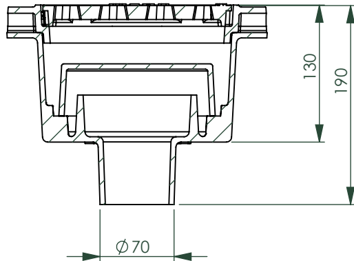
B-B (1 : 5)
