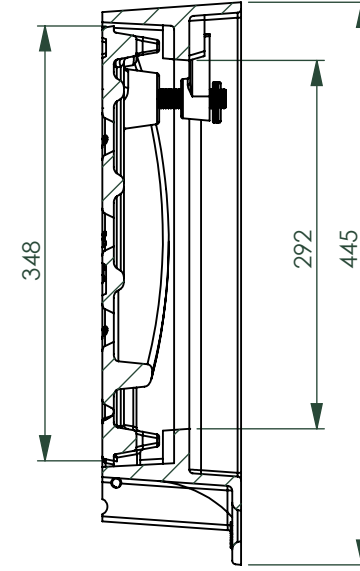
B-B (1 : 6)
