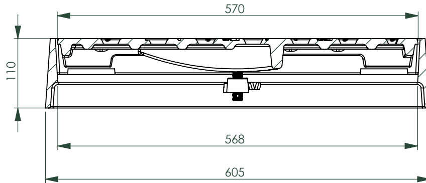
A-A (1 : 6)
