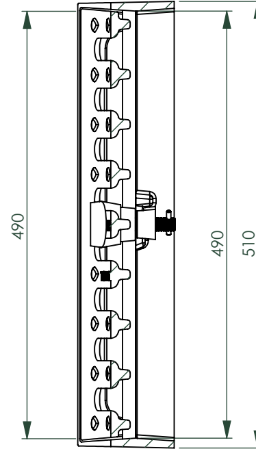
A-A (1 : 6)
