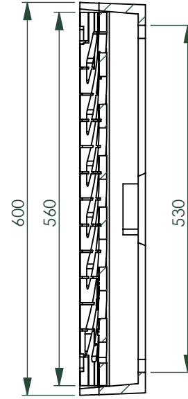
B-B (1 : 8)
