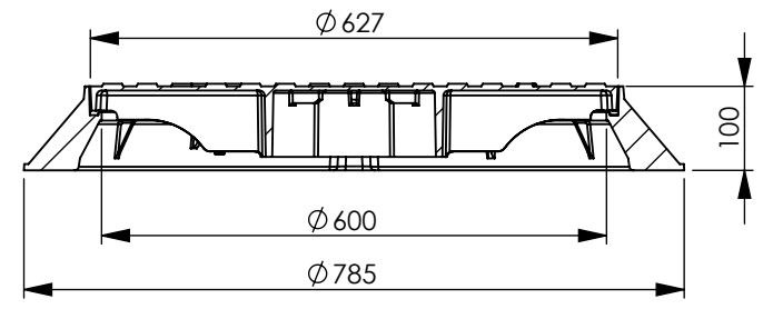
A-A
