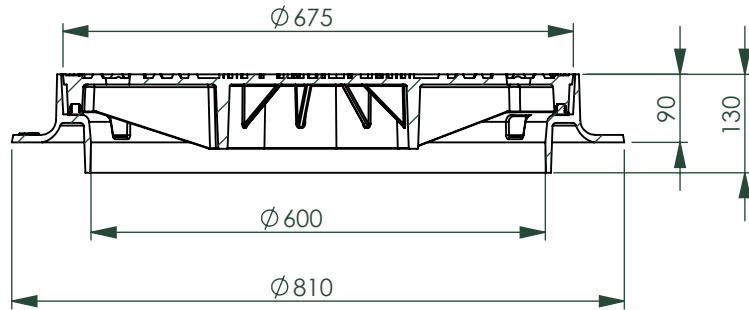
A-A (1 : 10)
