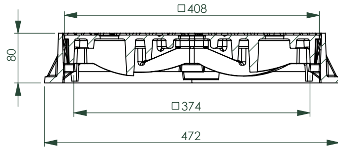
B-B (1 : 6)
