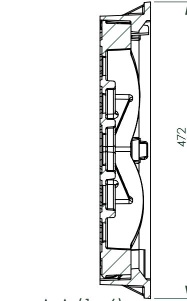
A-A (1 : 6)
