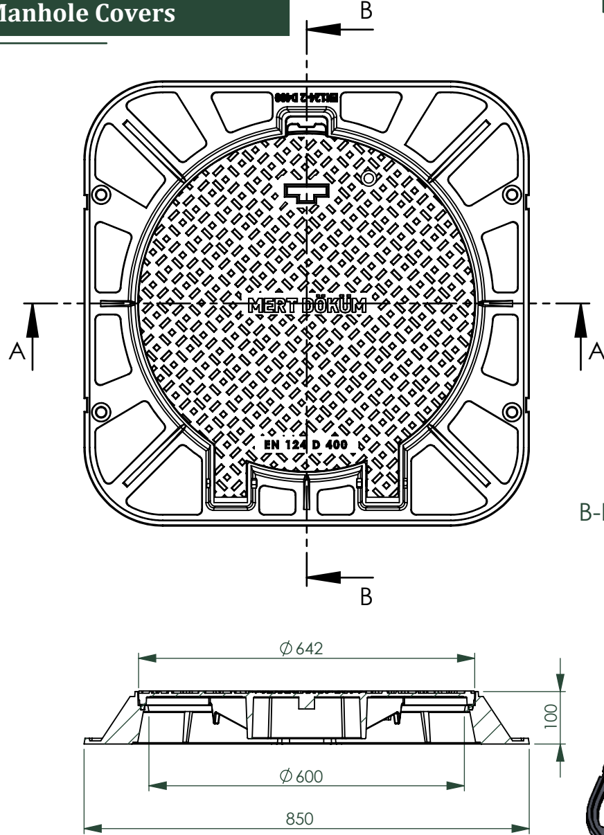
A-A (1 : 10)
