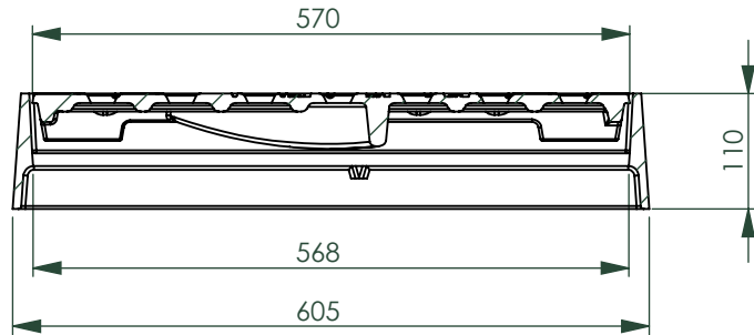
B-B (1 : 8)
