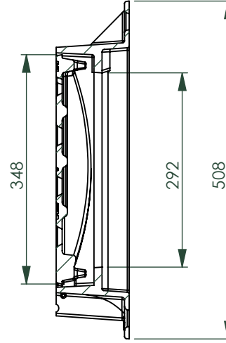
A-A (1 : 8)
