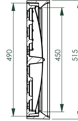
B-B
