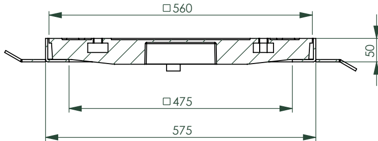
B-B (1 : 8)
