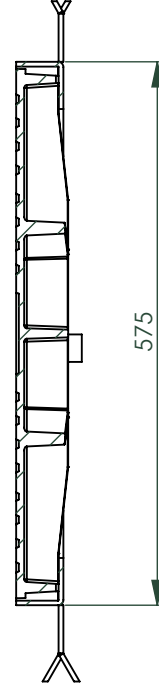
A-A (1 : 8)
