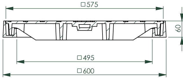
A-A (1 : 8)
