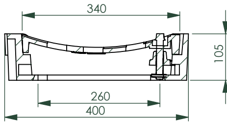
A-A (1 : 8)
